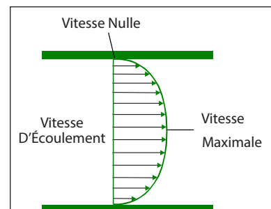
Figure 2. Profil de Vitesse
