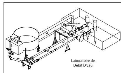
Figure 9. Installation de Calibrage 40k Gravimétrique
