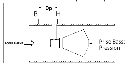
Figure 1. Prises Basse et Haute Pression
