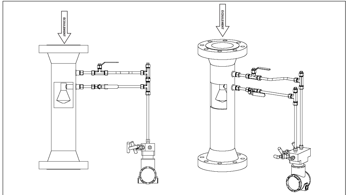
Figure 27. Installation sur Tuyauterie Verticale (Flux Descendant) pour une Application Impliquant un Liquide sans Air/Gaz Entraîné
