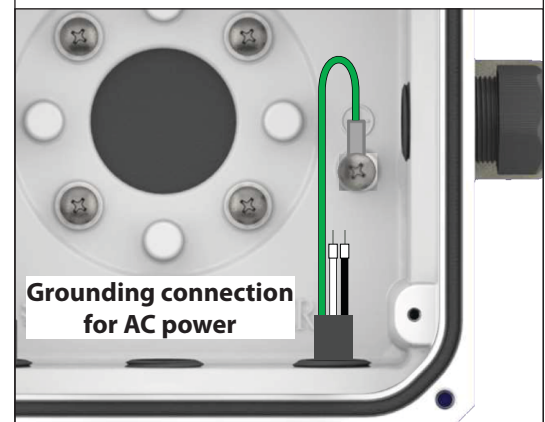
Grounding lug
